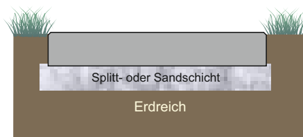
Einbauskizze:
