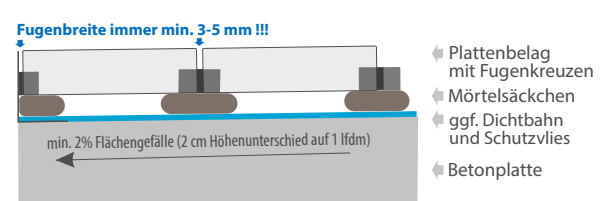
c) auf Zement-Mörtelsäckchen
