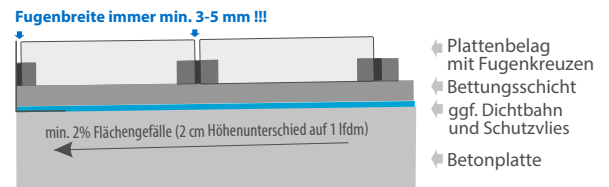
a) im Splittbett
