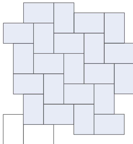
BS M145b (Fischgrätmuster)
